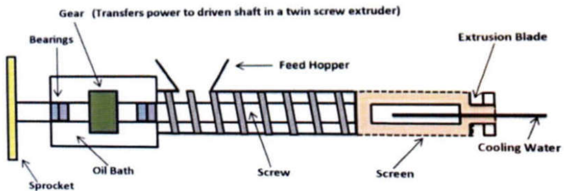
a. Extruder
